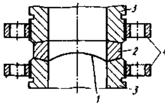
Рисунок 9.2 – Линзовый зажим разрывной мембраны: 1 – мембрана, 2 – коническая шайба, 3 – торцы сбросной магистрали, 4 – соединительные фланцы
