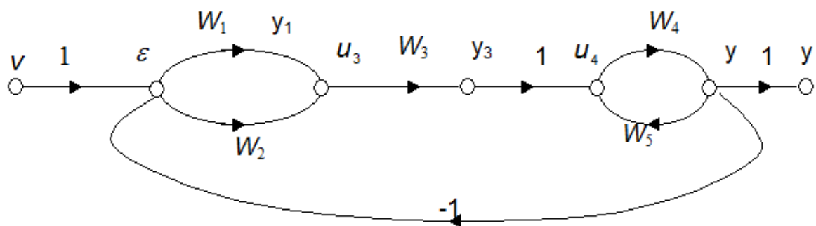
Рисунок 2 — Граф системы
