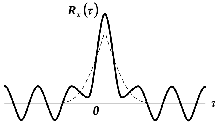
Рисунок 3 — Фильтрация полезного периодического сигнала с помощью его корреляционной функции
