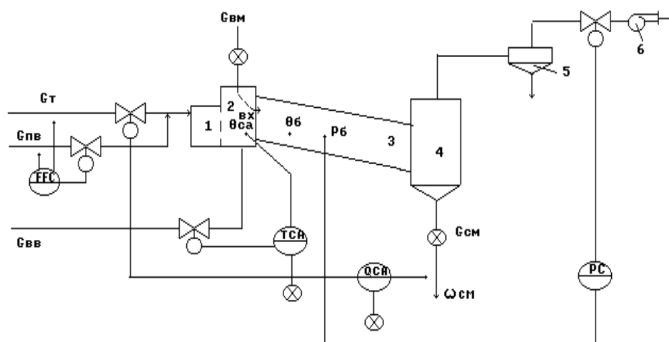
Рисунок А.8 – Схема автоматизации (б) барабанной сушилки прямо-точного действия (а):
