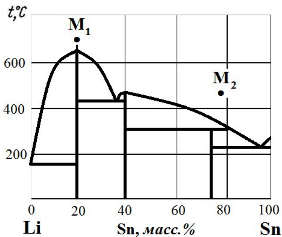
Рис.16. Диаграмма состояния Li – Sn.
