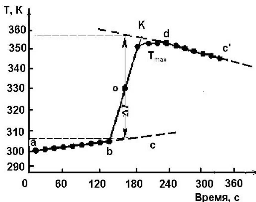
Рисунок 3.2 – Графическое определение \chi_T по методу Ланге-Мищенко
