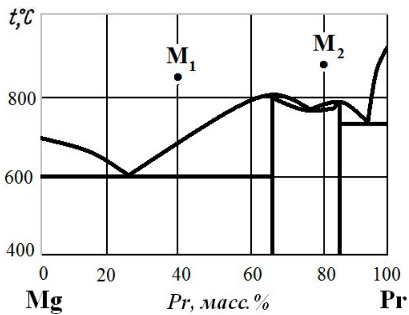
Рис.28. Диаграмма состояния Mg – Pr.
