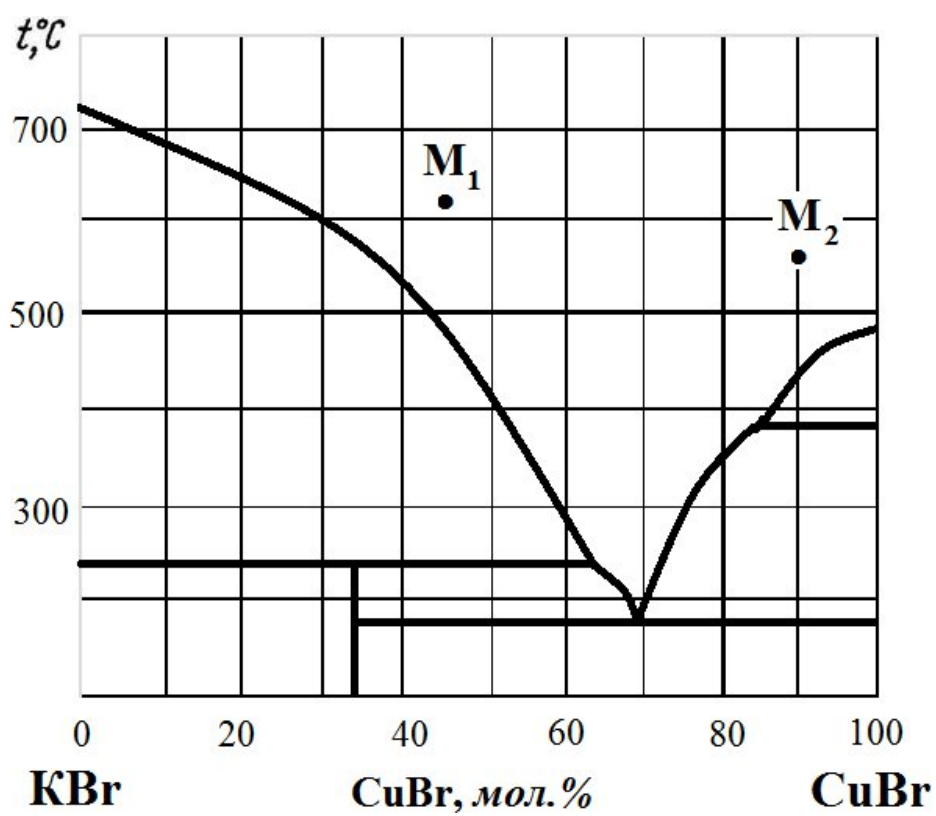
Рис.9. Диаграмма состояния KBr – CuBr.
