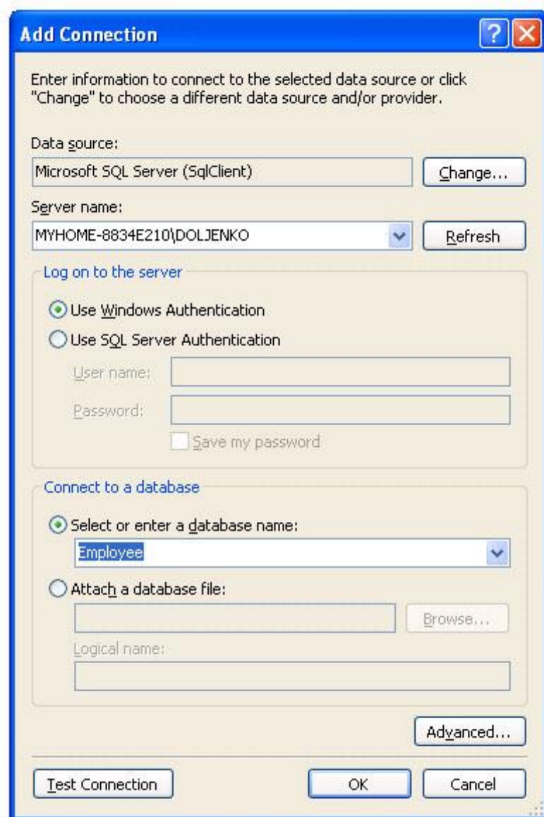
Рис. 8.5. Окно AddConnection
