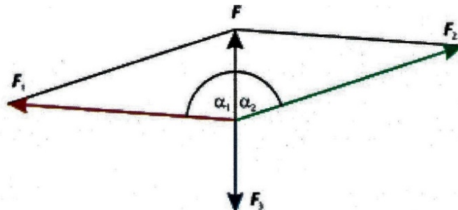
Рисунок 4.2 – Определение суммы векторов двух сил \mathbf{F}_1 и \mathbf{F}_2 по уравнивающей силе \mathbf{F}_3 .
