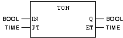
Рисунок 5 – Общий вид блока TON
