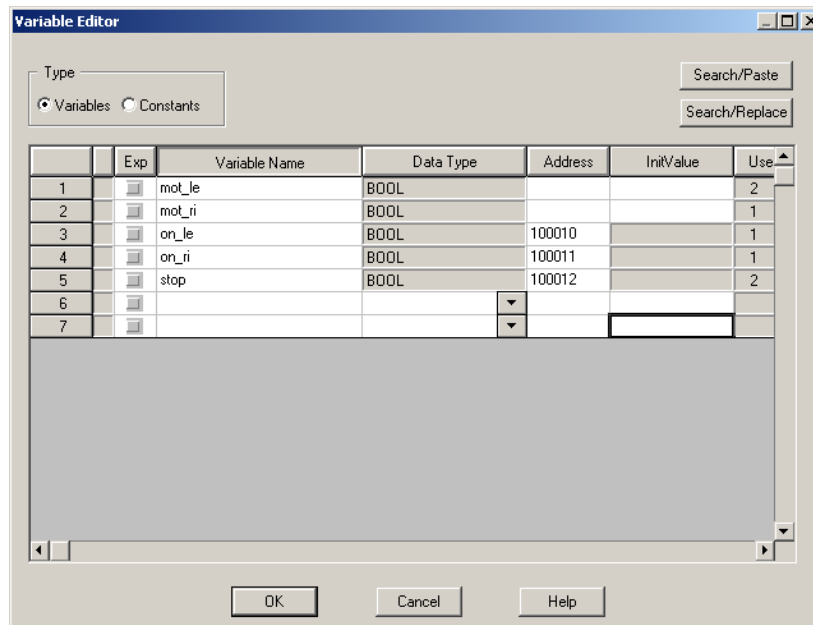
Рисунок 4 – Окно редактора переменных
