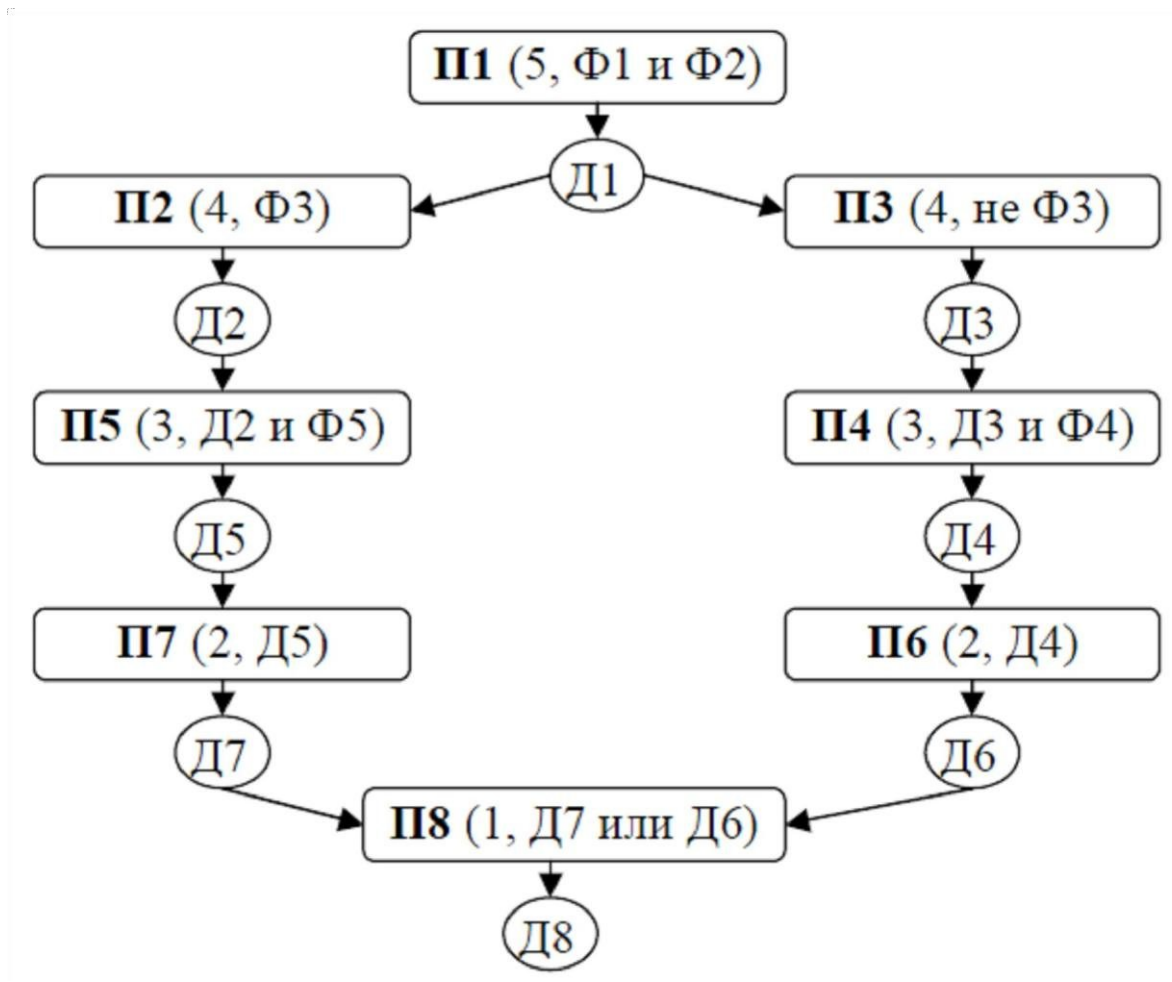
Рисунок 1 – Граф модели знаний
