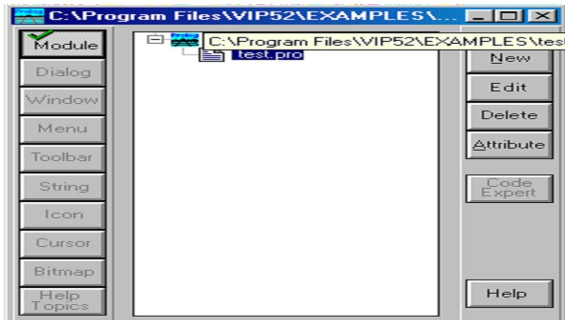
Рисунок 10 – Окно проекта
