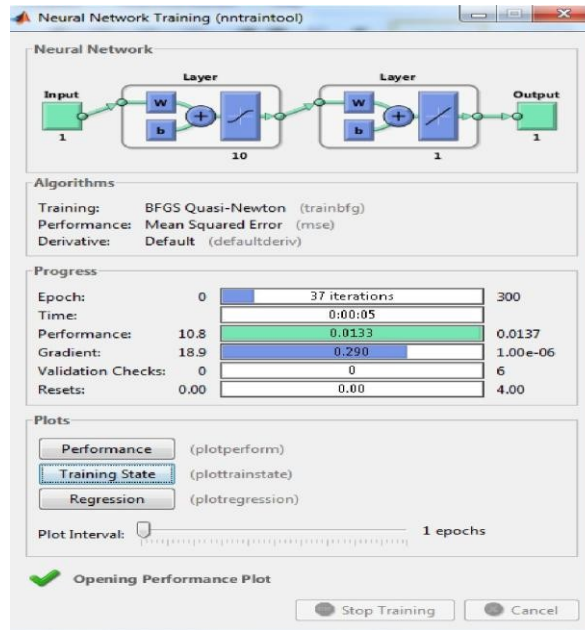
Рисунок 23 – Обучение сети
